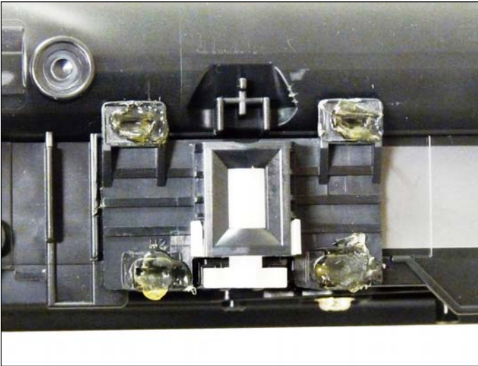
13. Coloque la cubierta del sello de nuevo y con pegamento caliente péguela. Si realizo los 4 agujeros, instale los cuatro tornillos auto ajustables.
