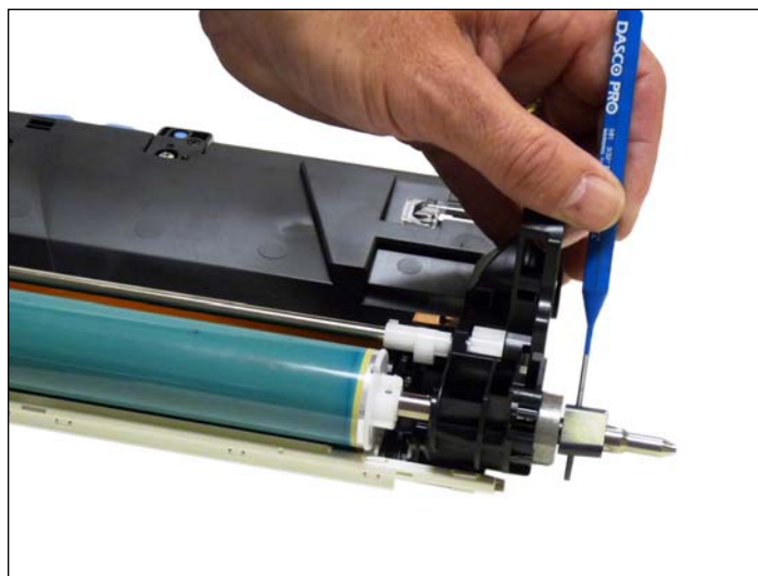
25. Saque el pin hacia afuera del eje de engranaje guía metálico del cilindro. Remueva el engranaje.
