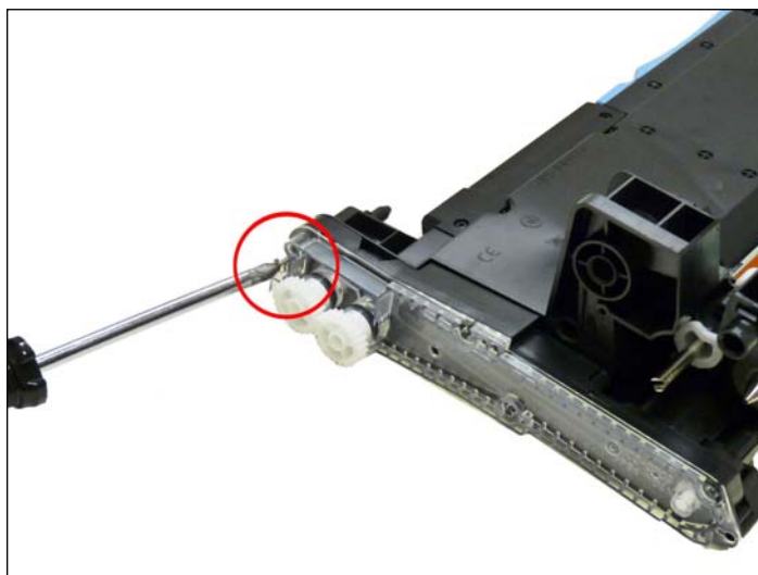
35. Instale el tornillo del ensamblaje del cinta/guía.
