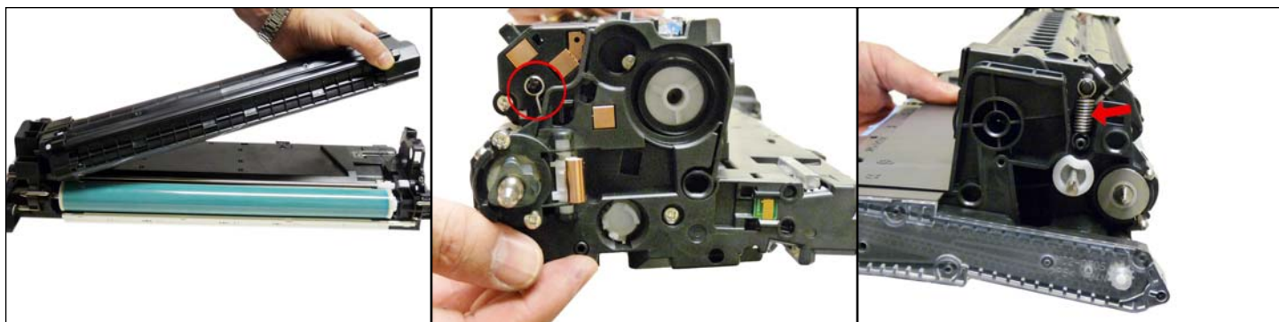
37. Instale la unidad del revelador en la unidad del cilindro.
