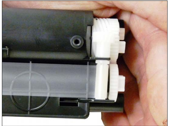
12. Instale el sello nuevo. Envuelva el sobrante en el engranaje superior.
