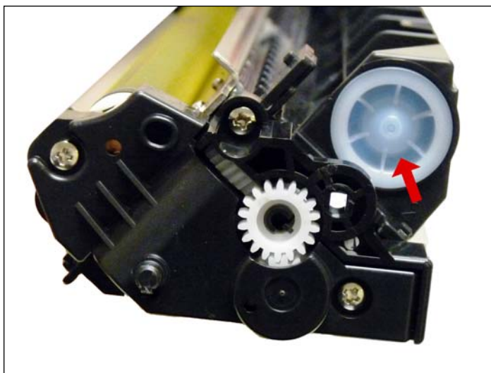
36. Cuando el rodillo revelador este disponible, remueva el tapón de llenado, saque el revelador antiguo, aspire la cámara e instale el rodillo revelador nuevo. En este momento no recomendamos que le haga nada a la cuchilla dosificadora.
