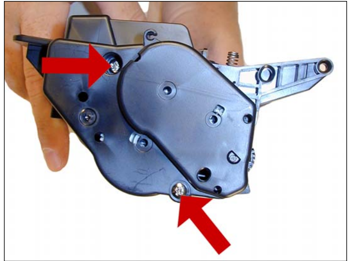
25. Instale la cubierta lateral con el engranaje y los dos tornillos. Si la cubierta lateral no puede ser colocada de manera correcta, quiere decir que el imán estacionario no está colocado adecuadamente.
