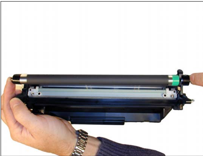
18. Remueva el ensamble del rodillo magnético del cartucho.
