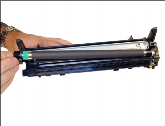
24. Limpie la manga del rodillo magnético con un limpiador dedicado para rodillos magnéticos. Instale el rodillo magnético. Gire el imán estacionario de manera que el extremo angulado entre en la cubierta lateral, no podrá ver el extremo angulado así que tendrá que colocar el imán sintiéndolo mientras lo gira
