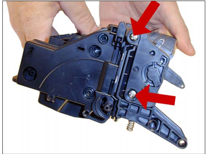
23. Instale la cubierta lateral y los dos tornillos.
