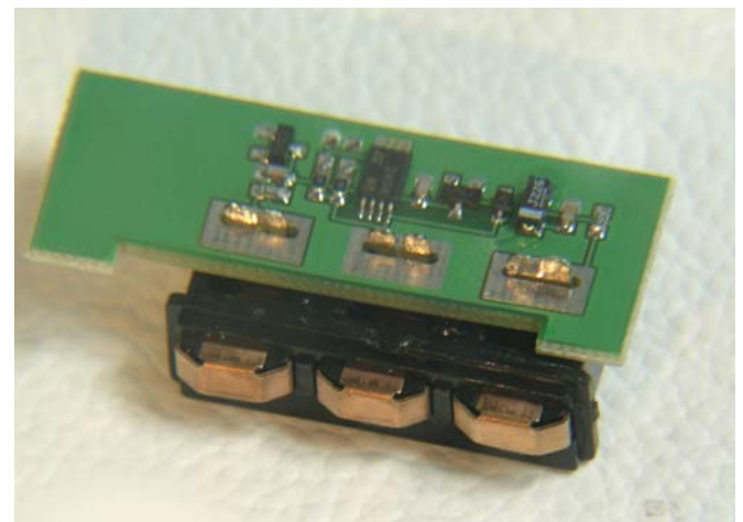
CHIP DE REEMPLAZO (MONTADO EN SU CONECTOR) VER PAGINA 5
