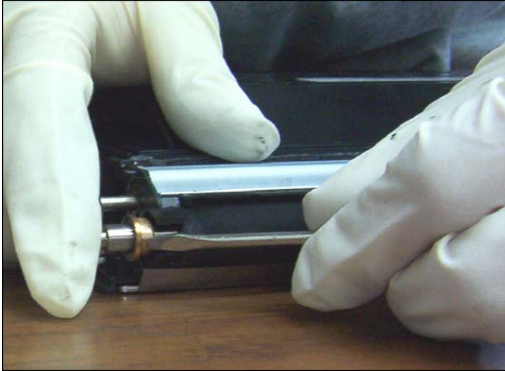
7. Sacar el buje metálico que mantiene el eje en su lugar cerca de donde el tapón de llenado de toner esta ubicado. El buje opuesto puede permanecer en su lugar.
