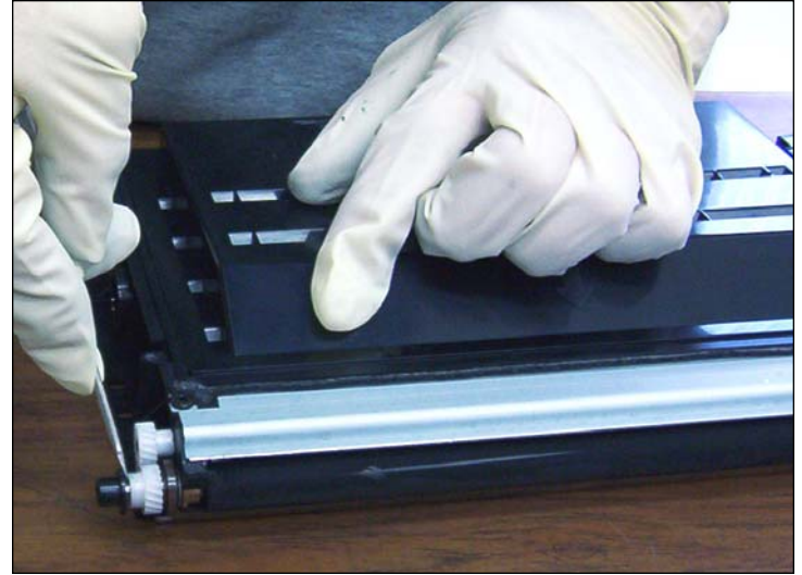
6. Sacar el clip metálico con ayuda de un pequeño desarmador plano. Sacar el clip hacia arriba para apartarlo del eje.
